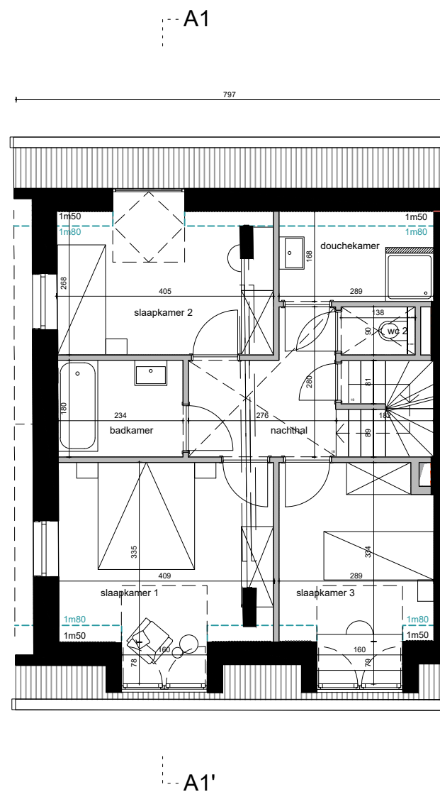
NIVEAU +1
