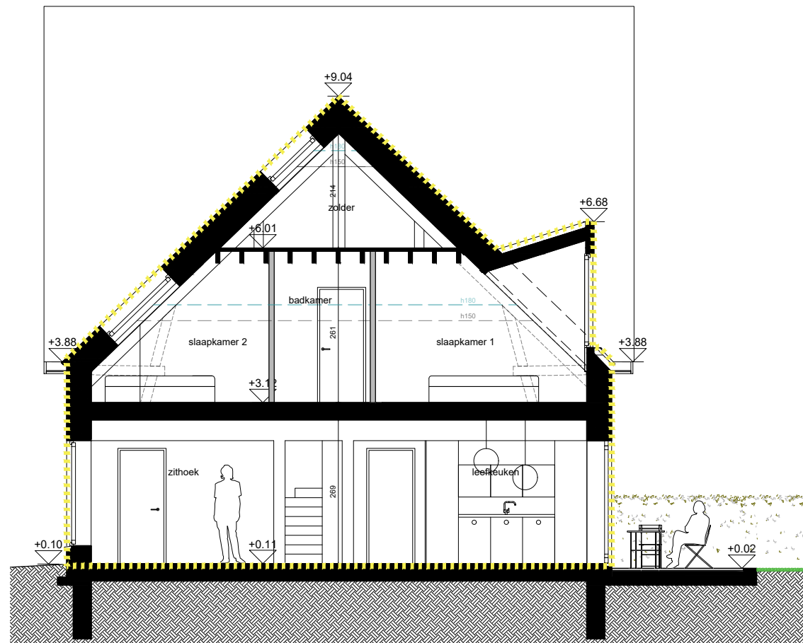
SNEDE A1
