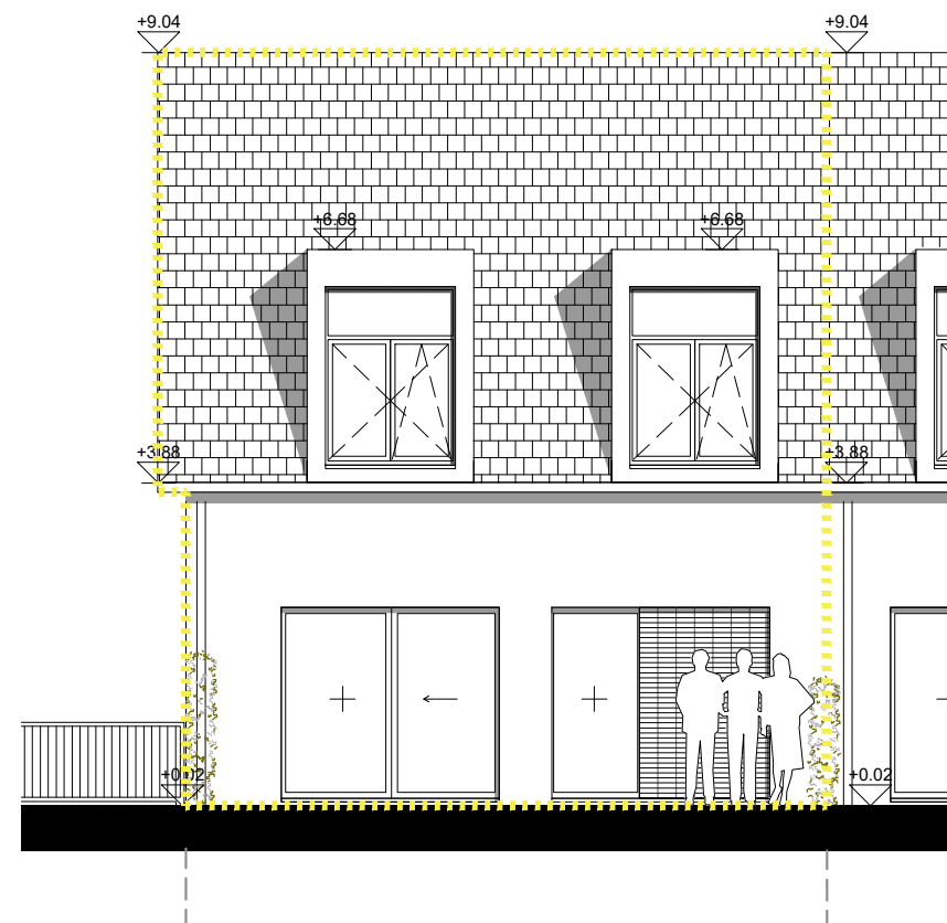
ZUID GEVEL
