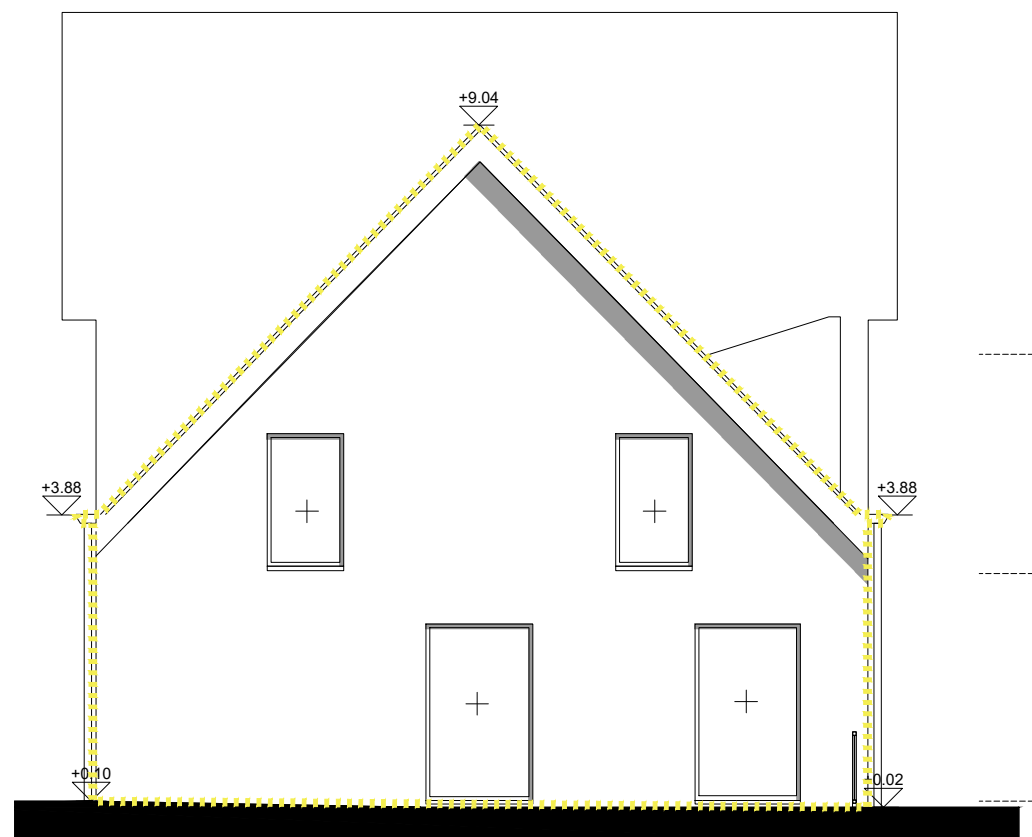
WEST GEVEL
