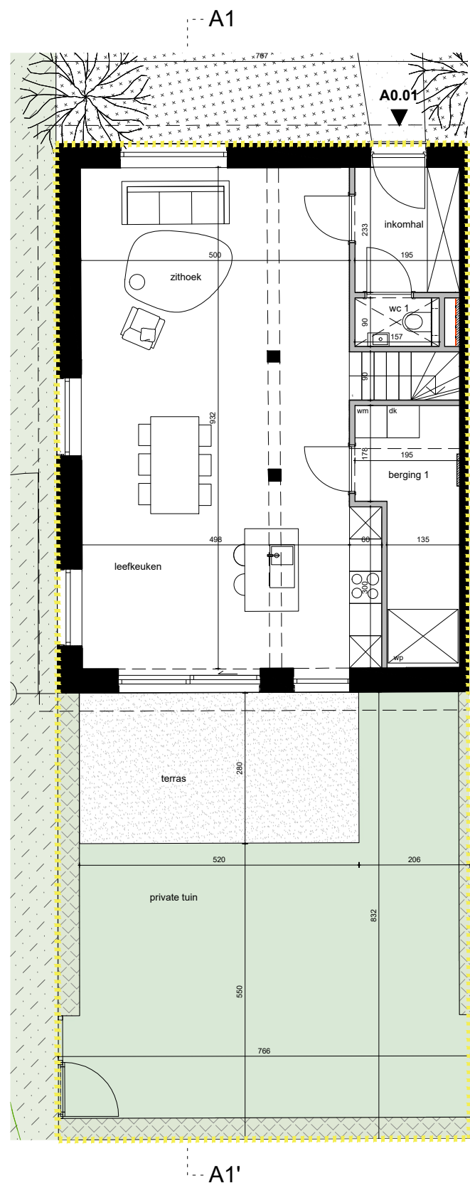
NIVEAU 0
