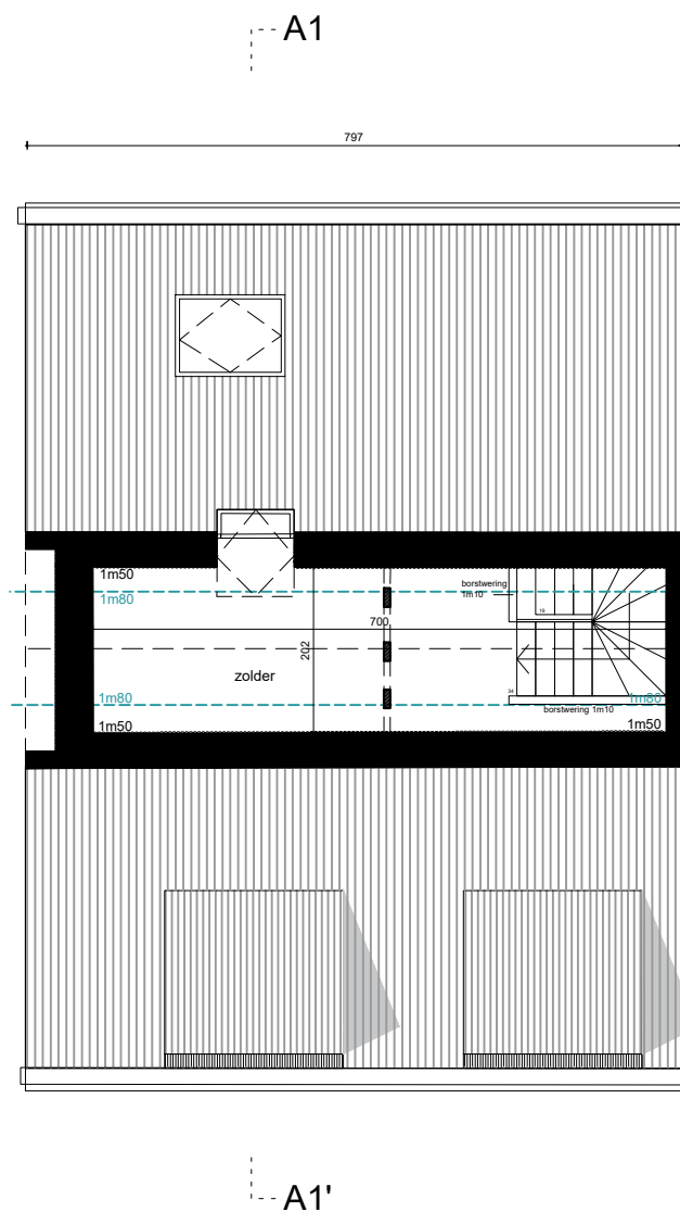
NIVEAU +2
